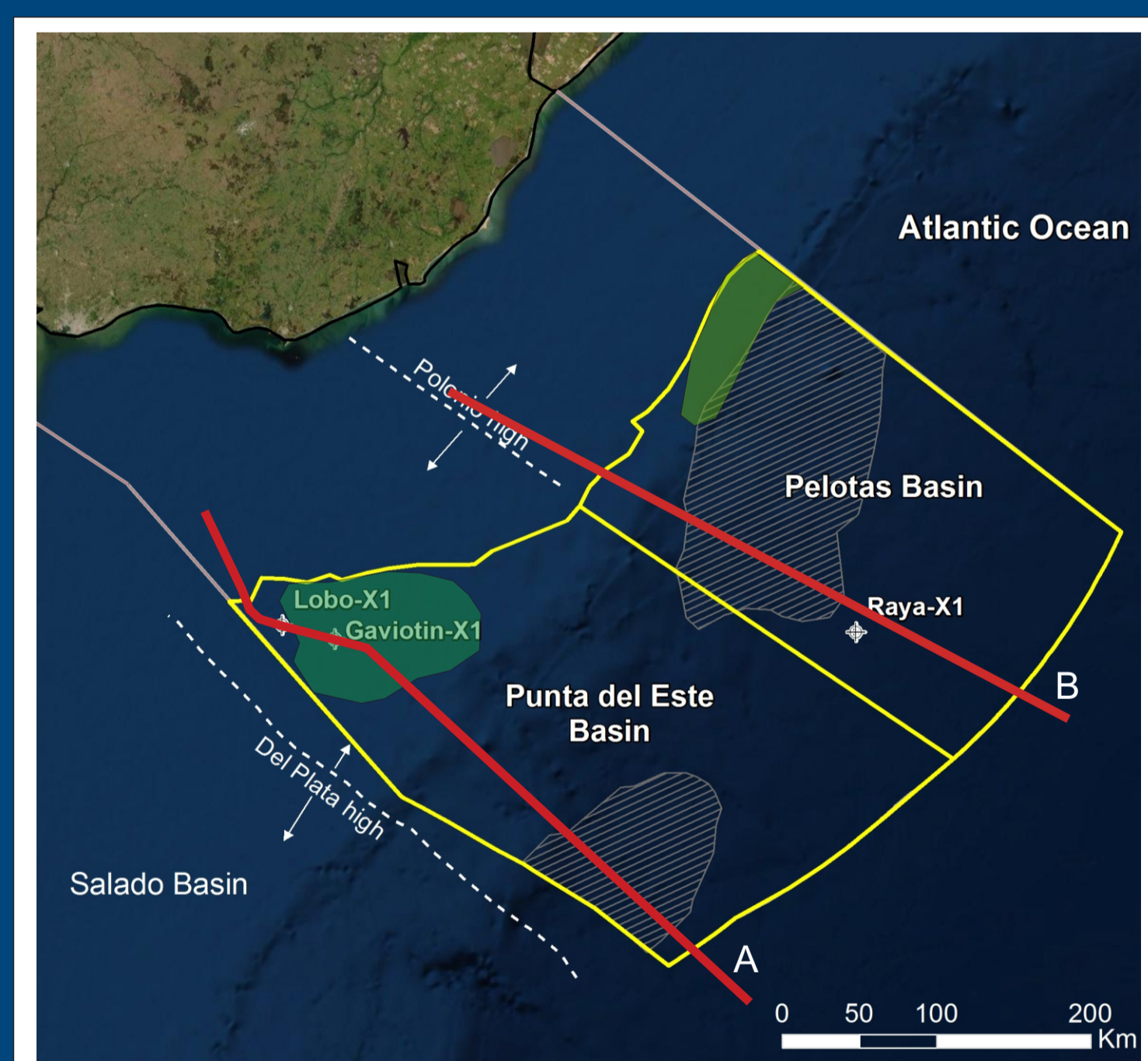
Prerift source rock
