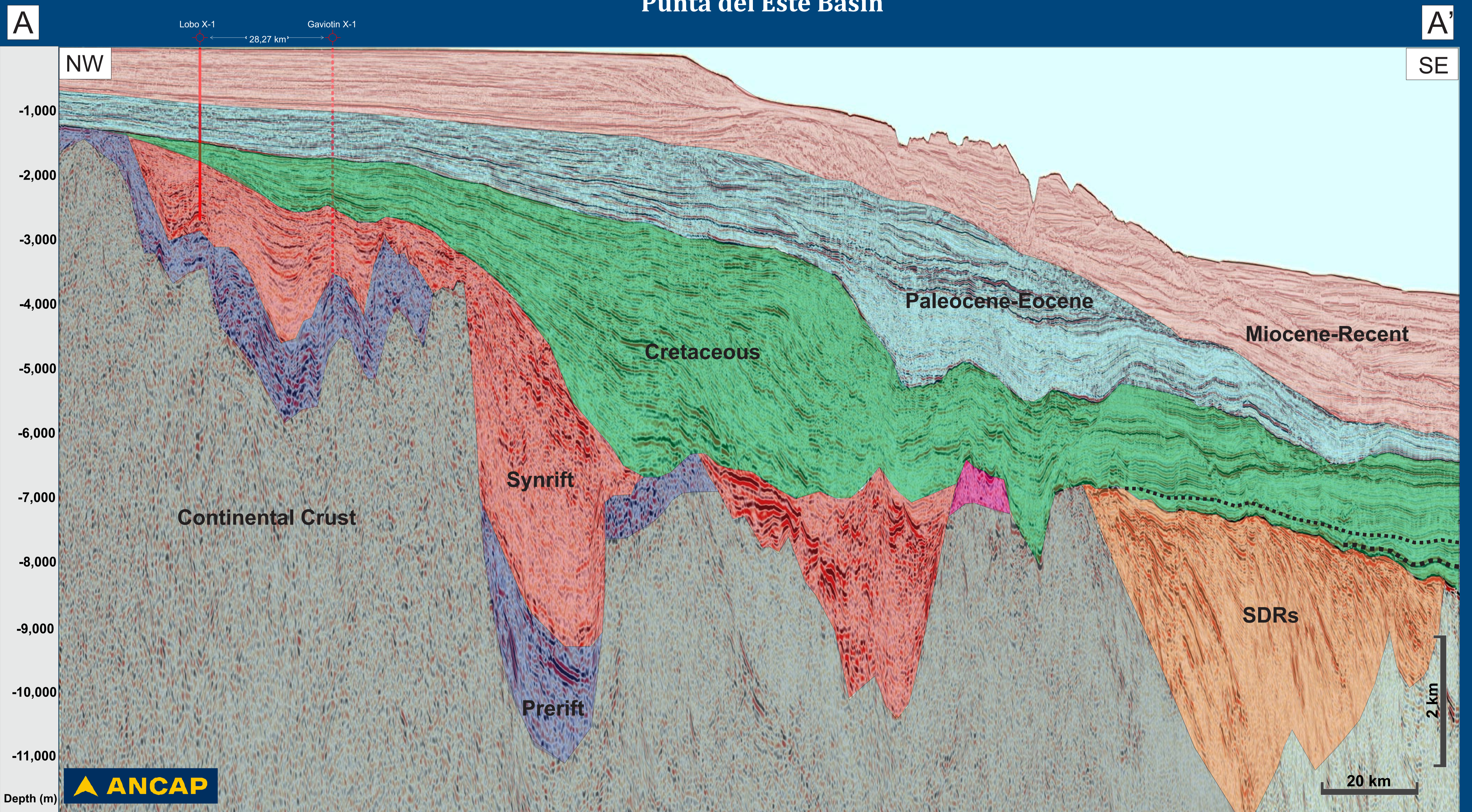
Punta del Este Basin
