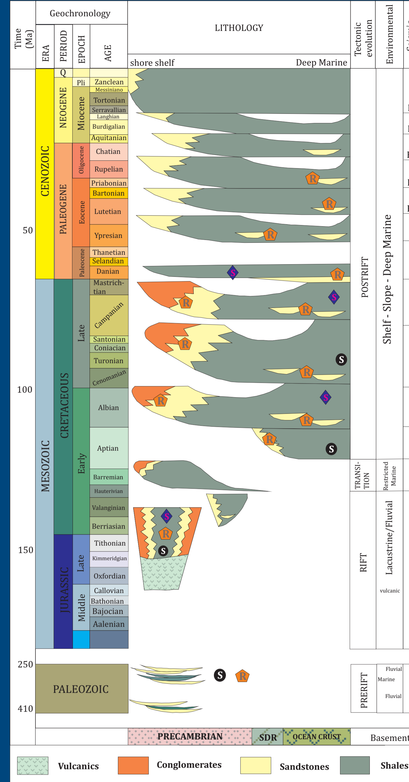
Punta del Este Basin
